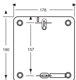
用户报警主机安装尺寸
